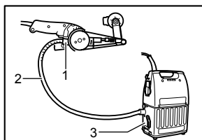
1. Buse 2. Tuyau 19 3. Collecteur de poussière
